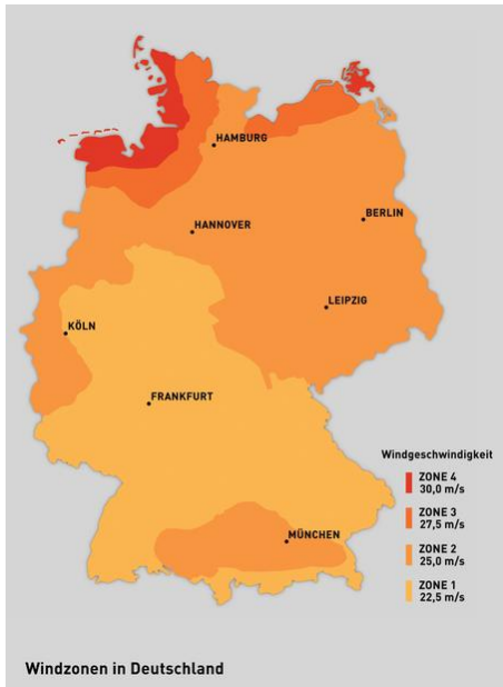
Abb. 25: Bereiche der Windzonen 1 bis 4 mit den zugehörigen Windgeschwindigkeiten (Quelle: Bundesamt für Bevölkerungsschutz und Katastrophenhilfe BBK)
